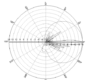
2140 MHz
